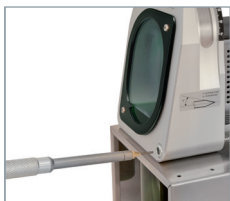
Præcis længdebestemmelse af elektrodens stick-out
